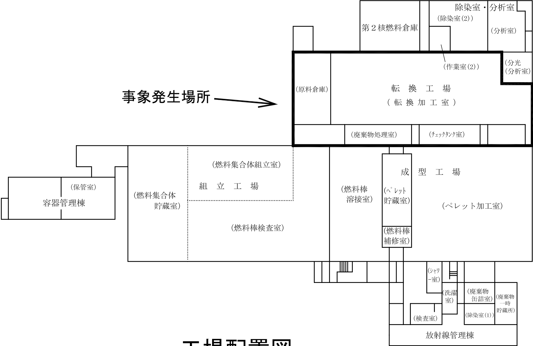
工場配置図
